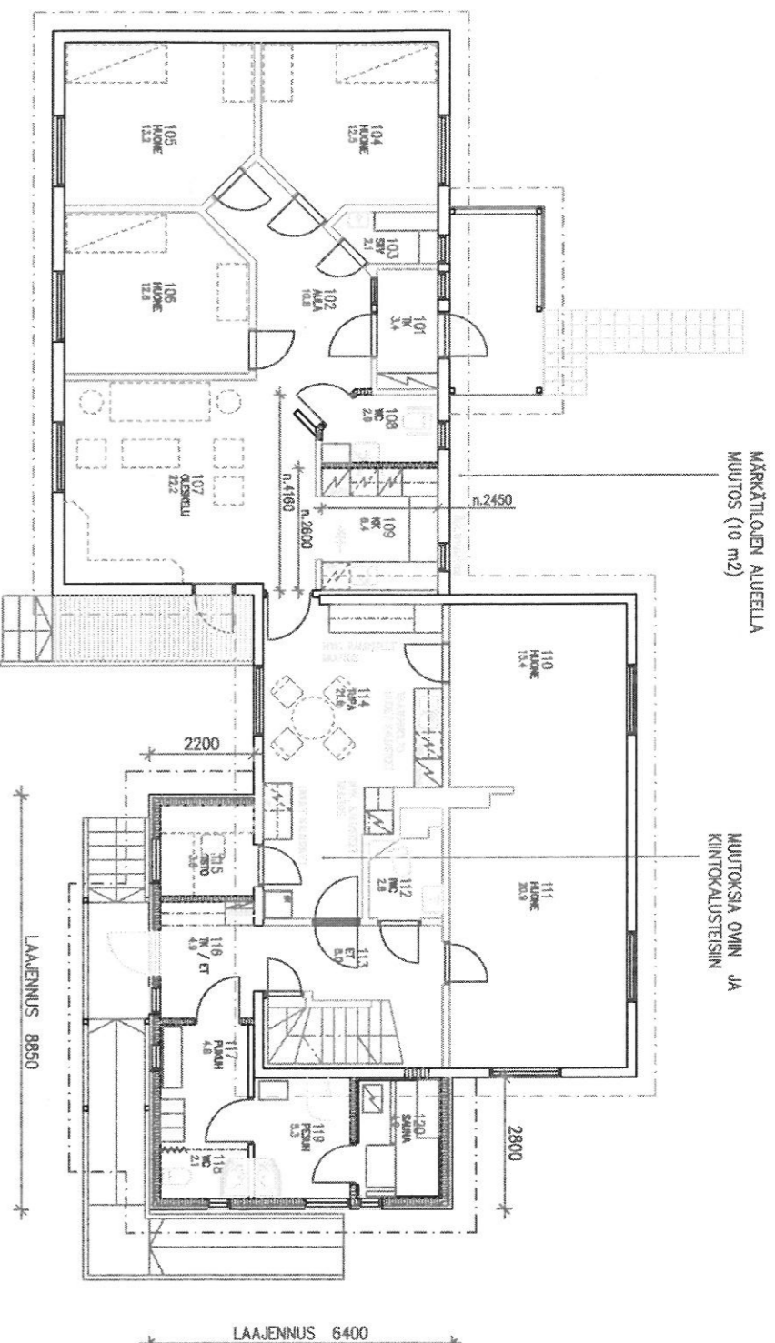
POHJA 1:100
