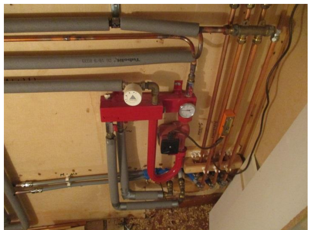
30. Portaikon putkia
