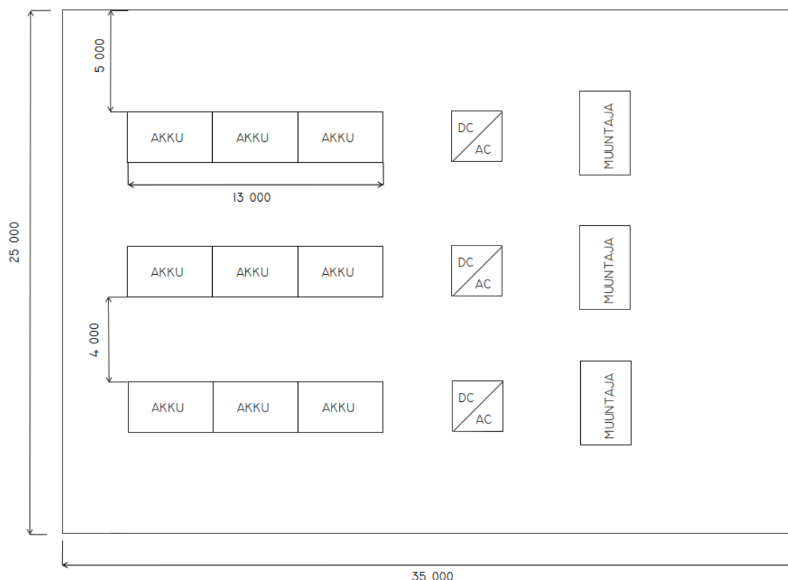
Kuva 2-15. Sähköenergiavaraston (10 MW) periaatekuva.
