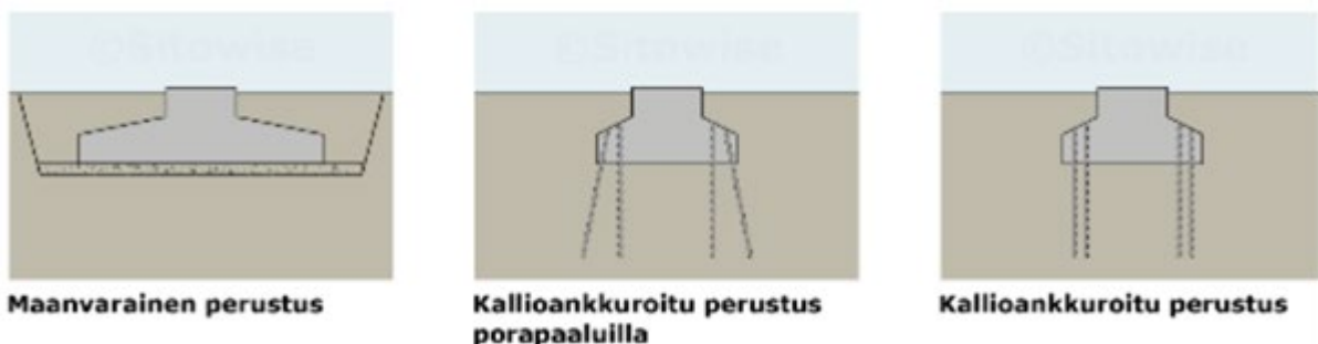
Kuva 2-7. Tuulivoimaloiden perustamistekniikoita.
