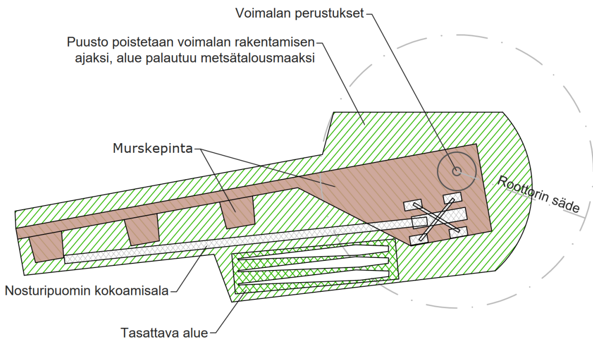
Kuva 2-8. Periaatekuva pinnoitettavasta nostoalueesta ja alueesta jolta puusto poistetaan.
