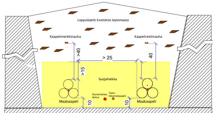
Kuva 2-13. Kaapelikaivannon poikkileikkaus.
