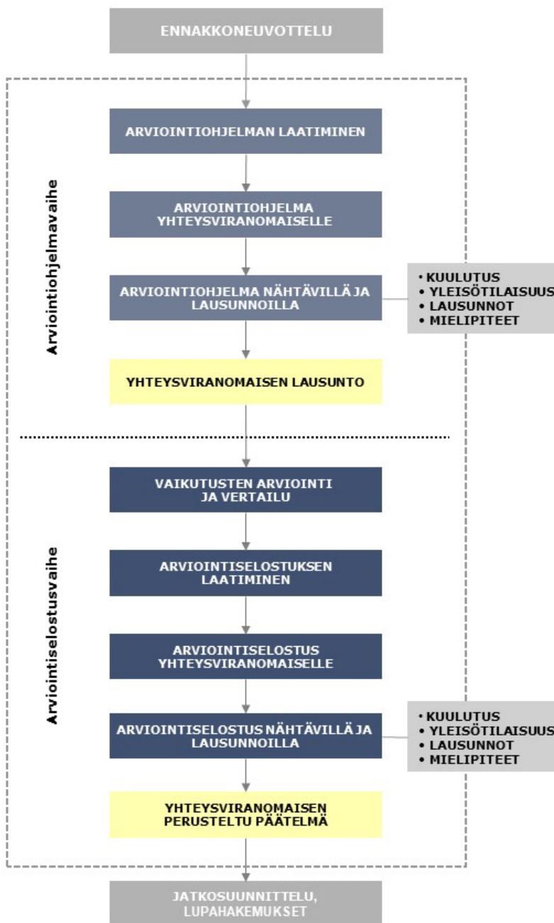
Kuva 3-1. YVA-menettelyn vaiheet.
